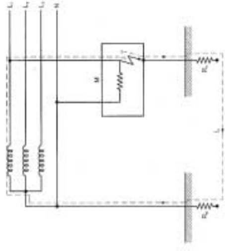
Figura 4 Esquema TT
