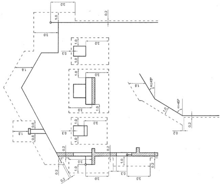
Figura 1. Zona de protección en edificios para la instalación de líneas eléctricas de baja tensión con conductores desnudos.
